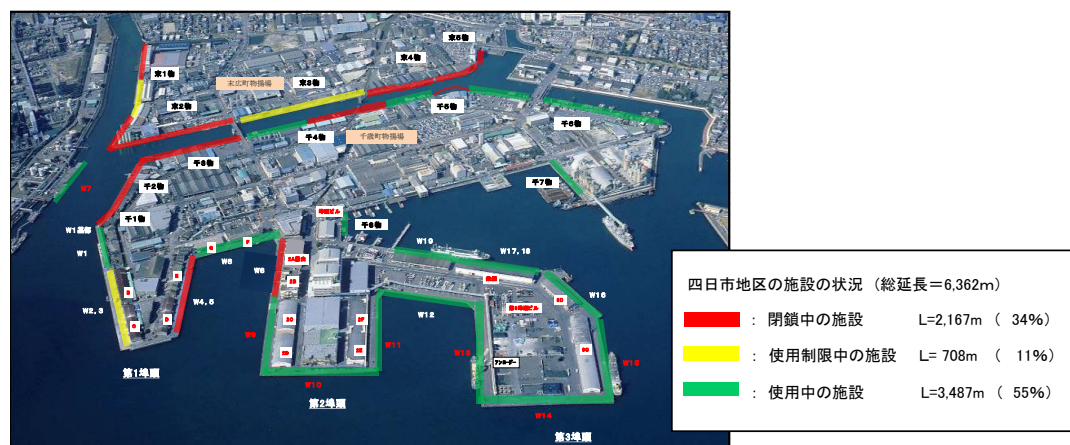
図 5-3-2 四日市地区における港湾施設の状況
