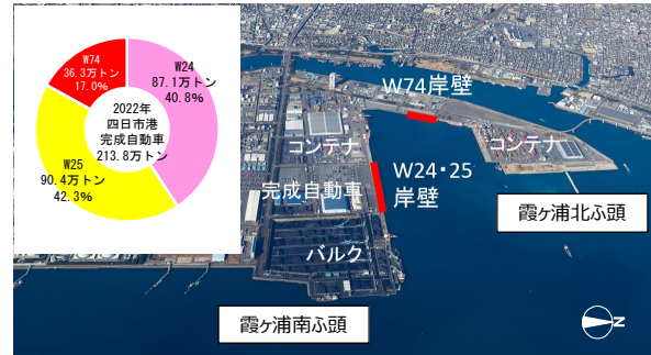
図 1-4-8 四日市港の完成自動車の取扱ベース (*)
