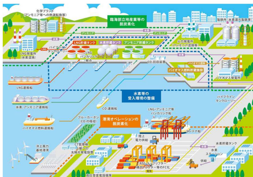
図 1-8-1 カーボンニュートラルポート(CNP)の形成イメージ
